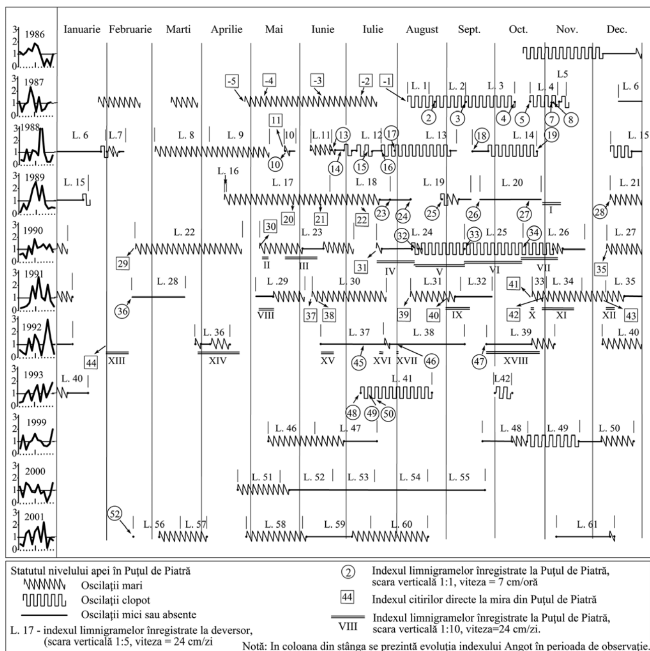
Fig. 10.5. Sinteza observațiilor efectuate asupra oscilațiilor nivelului apei în Puțul de Piatră.
