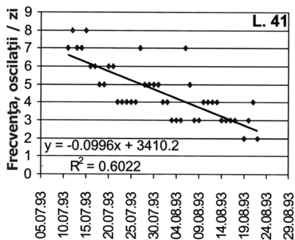
Fig. 10.14. Reducerea în timp a frecvenței oscilațiile clopot.
