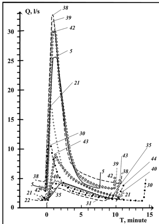
Fig. 10.7. Forma oscilațiilor mari din Puțul de Piatră (stânga) și evoluția debitului izbului pe durata acestor oscilații (dreapta).
