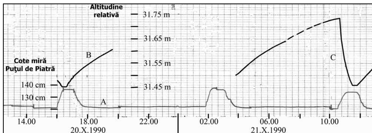
Fig. 10.18. Măsurători simultane ale variației nivelului apei în Puțul de Piatră (A) și în lacul din avenul din valea Vulpilor (B și C), efectuate la 20-21 octombrie 1990.
