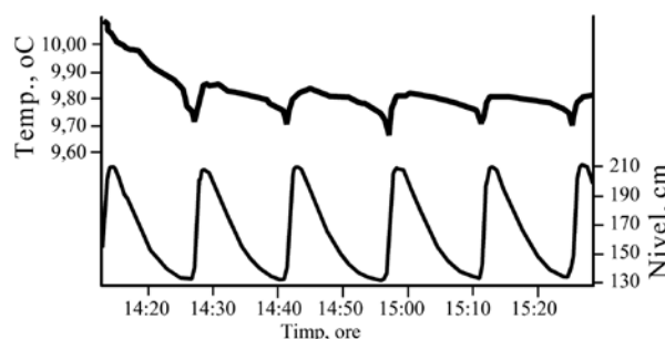
Fig. 10.6. Evoluția nivelului și temperaturii apei izbului pe parcursul oscilațiilor mari înregistrate la 25 noiembrie 2004 cu ajutorul unui senzor.
