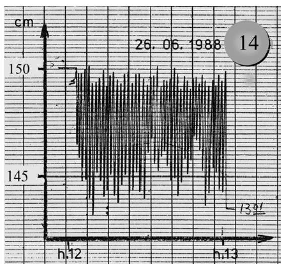
Fig. 10.11. Oprirea oscilațiilor mari
