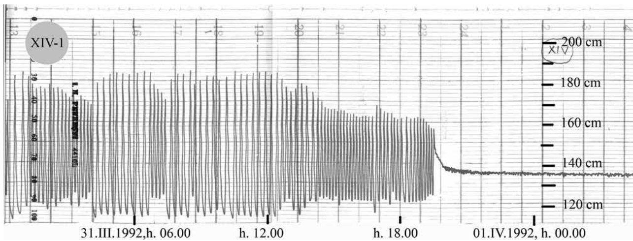
Fig. 10.11. Oprirea oscilațiilor mari
