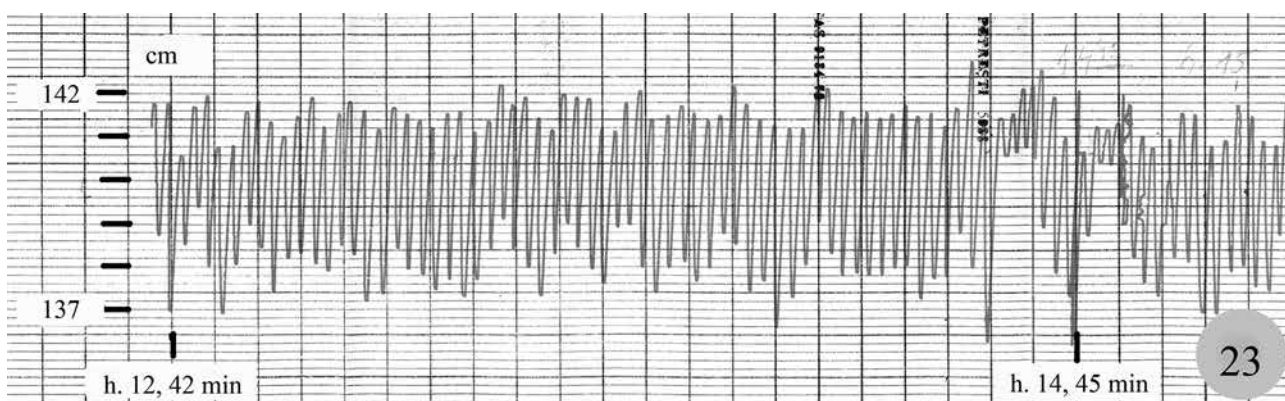
Fig. 10.12. Diferite forme ale oscilațiilor mici.
