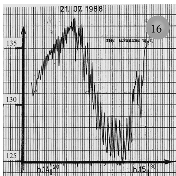
Fig. 10.12. Diferite forme ale oscilațiilor mici.
