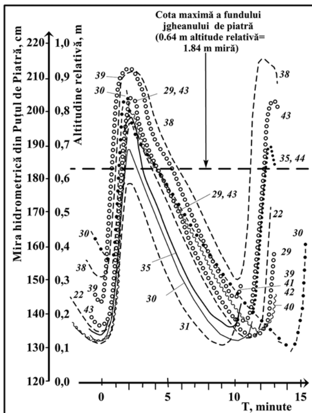
Fig. 10.7. Forma oscilațiilor mari din Puțul de Piatră (stânga) și evoluția debitului izbului pe durata acestor oscilații (dreapta).
