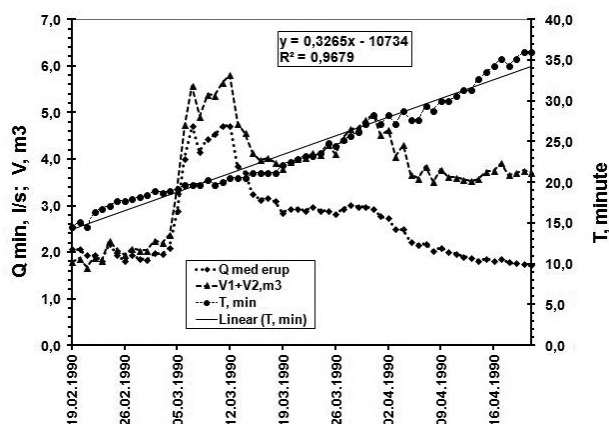
Fig. 10.10. Rezultatele prelucrării limnigranei L. 22 înregistrată la deversorul izburului în perioada 18.02-25.04. 1990.
