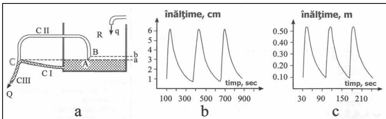
Fig. 10.22. Modelul propus de Mangin (a), a generat oscilații ale nivelului apei (b), identice cu cele înregistrate la izvorul Fontestorbes (c).
