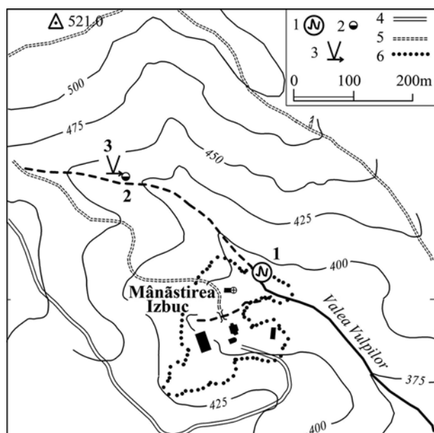
Fig. 10.3. Plan cu amplasamentul izbucului.
