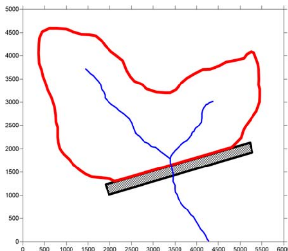
Fig.5. Bazinul hidrografic al secțiunii barajului
