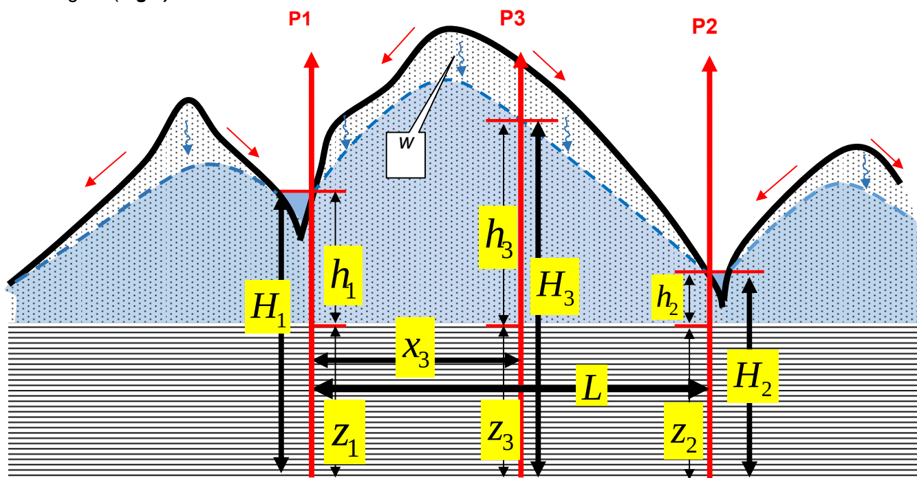
Fig.2. Secțiune pentru calculul modulului de infiltrare ( w )
