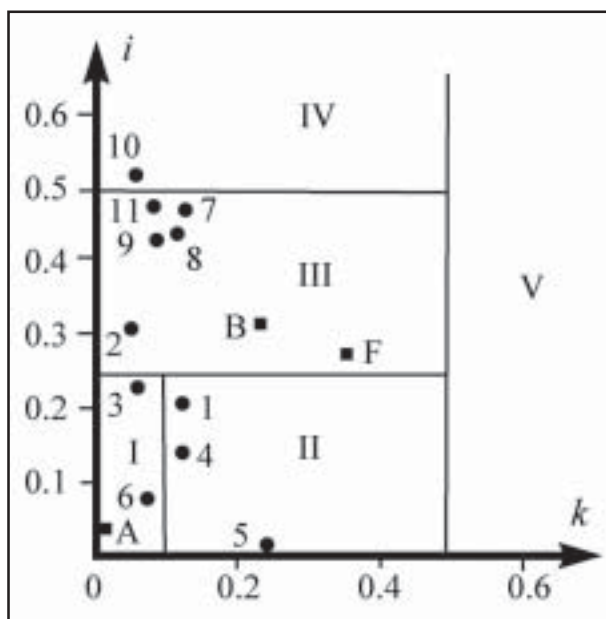
Figure 2.5. Position of major karst system according to Mangin's classification (1975): 1 - Aștileu, 2 - Brătcani, 3 - Izbândiș, 4 - Toplița de Vida, 5 - Toplița de Roșia, 6 - Roșia (Pădurea Craiului Mountains), 7 - Păuleasa, 8 - Tăuz (Bihor Mountains), 9 - Boiu, 10 - Șopoteaș, 11 - Grota Ursului (Codru Moma Mountains)
